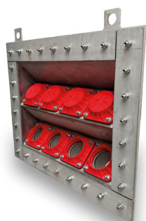
KRASO® Kabeldurchführung KDS 150 FL/ZE als Mehrfachdichtpackung - 45 Grad, Zum Einbetonieren (Sonderanfertigung)
